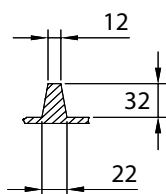
Tværsnit A-A
