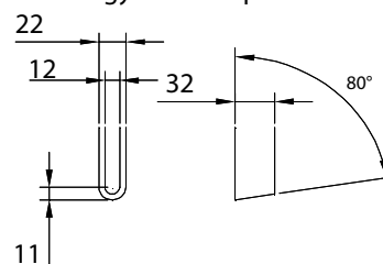
Profiludformning C-C begyndelse af profil
