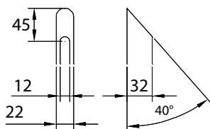
Profiludformning B-B begyndelse af profil
