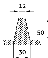
Tværsnit A-A
