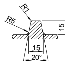
Profiludformning B-B
