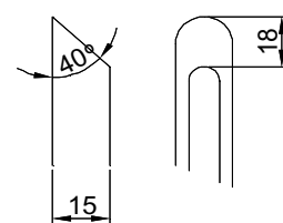
Profiludformning
