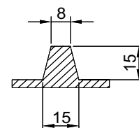
Tværsnit A-A
