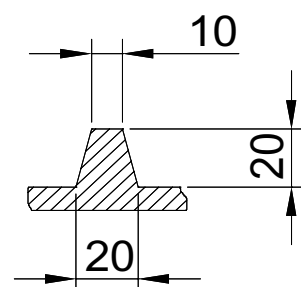
Tværsnit A-A
