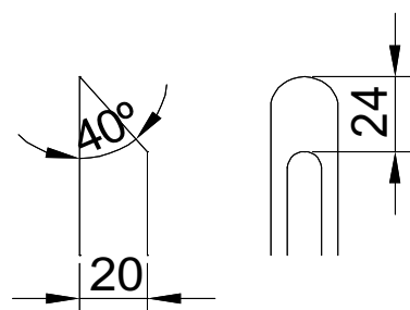
Profiludformning B-B
